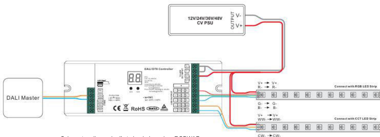
Schemat podłączenia dla trybu: jeden adres RGBWAF
