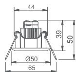
Głowica LED okrągła 100 / Round LED head 100
